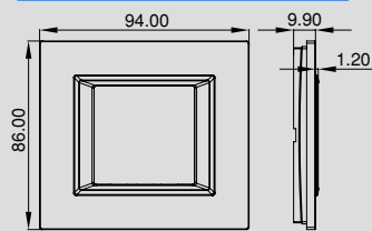
Ultima 2M Frame
