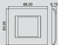
Sistema 2M Frame
