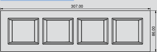
Ultima 4x2M Frame
