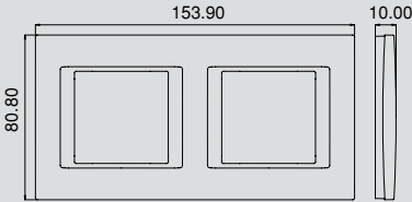
Optima 2x2M Frame
