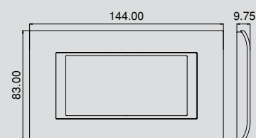
Sistema 4M Frame
