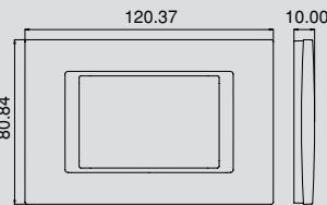
Optima 3M Frame
