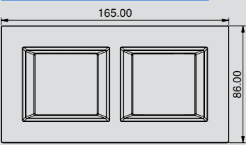
Ultima 2x2M Frame
