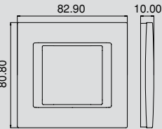
Optima 2M Frame
