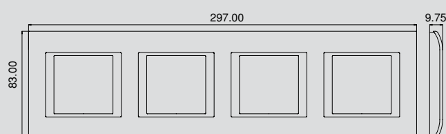
Sistema 4x2M Frame
